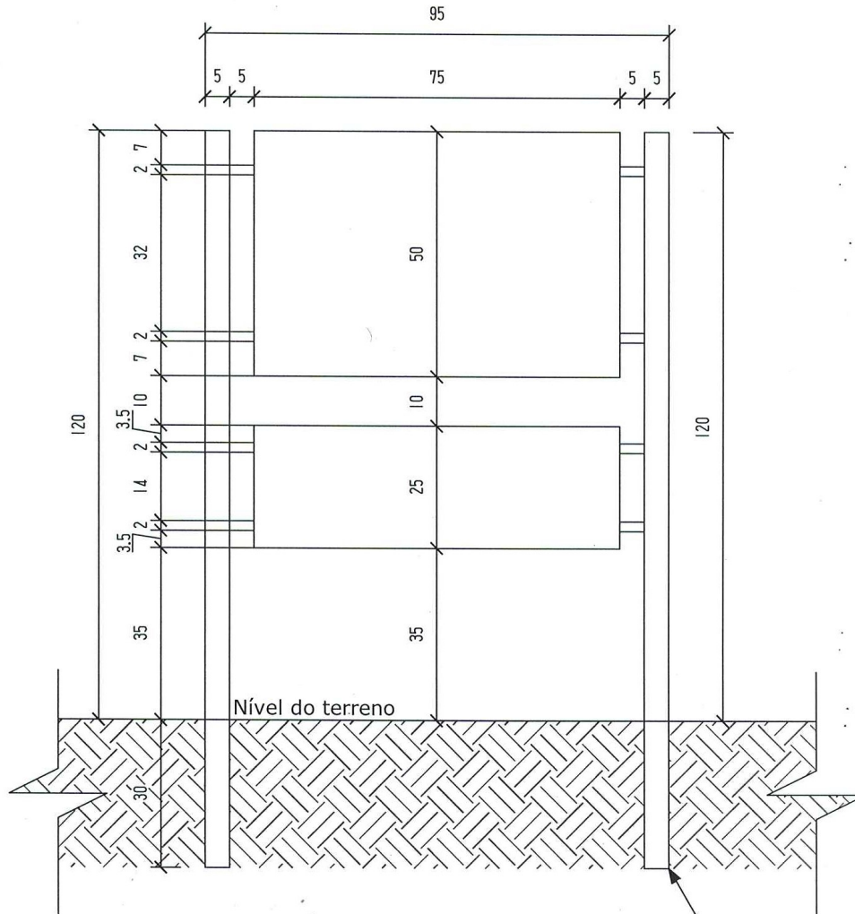
ELEVAÇÃO FRONTAL
